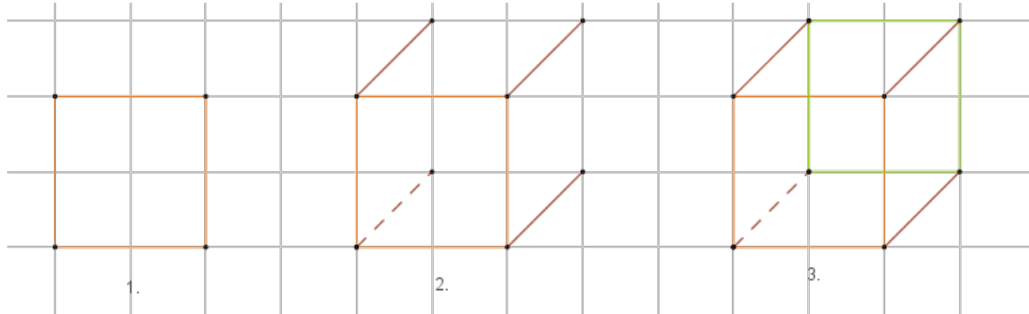
Abb. 1: Vorgehen zum Zeichnen eines Schrägbildes.
